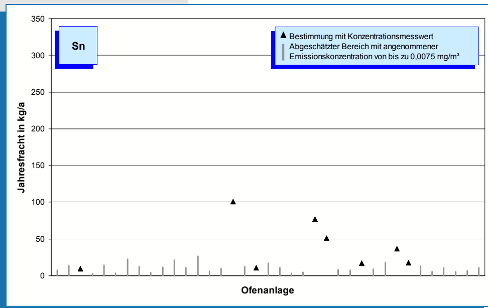
Bild 5-50: Zinn-Emissionen (Jahresfracht 2010) von 37 Drehofenanlagen.
