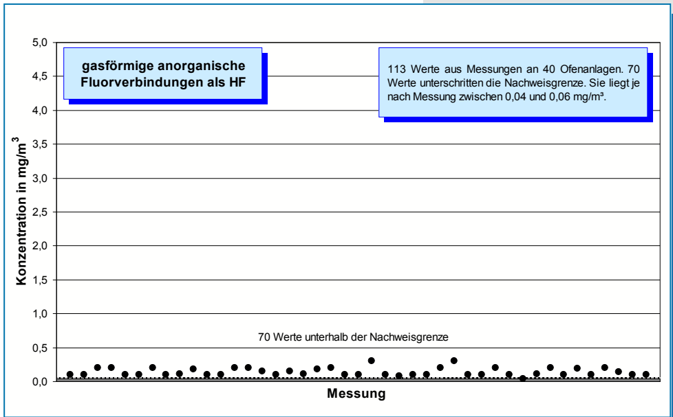
Bild 5-23: Messwerte (Jahr 2010) der Konzentration gasförmiger anorganischer Fluorverbindungen, berechnet als HF, im Reingas von 40 Drehhofenanlagen.
