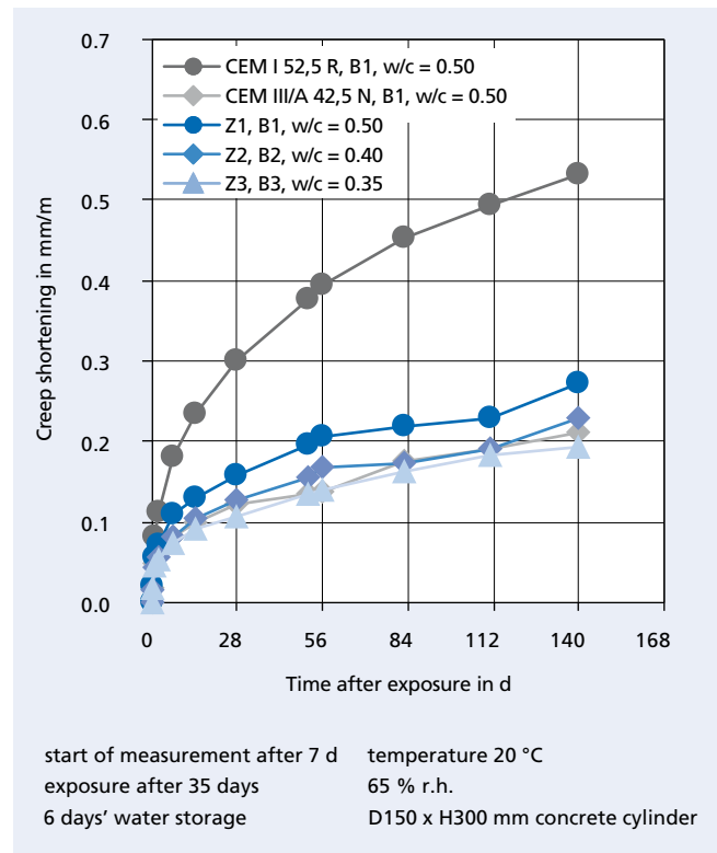
Bild 12: Kriechverformungen der Referenzbetone und der Betone mit klinkereffizienten Zementen Figure 12: Creep deformation of the reference concretes and of the concretes made with clinker-efficient cements
