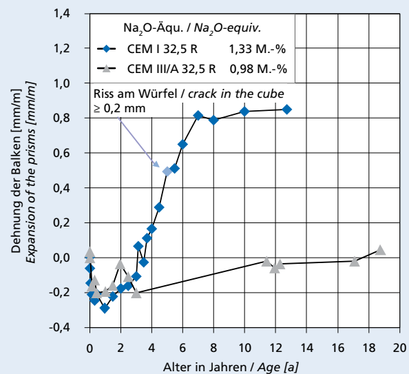
Bild 3: Dehnung eines Betons mit präkambrischer Grauwacke der Alkaliempfindlichkeitsklasse E III-S mit verschiedenen Zementen im Freilager. z = 500 kg/m 3 , w/z = 0,45, 30 Vol.-% Sand 0/2, 70 Vol.-% präkambrische Grauwacke E III-S 2/16 Figure 3: Expansion of a concrete composition made with crushed precambrian greywacke of the E III-S alkali reactivity class and various cements, stored in the outdoor exposure site. c = 500 kg/m 3 , w/c = 0.45, 30 vol. % sand 0/2, 70 vol. % crushed precambrian greywacke E III-S 2/16
